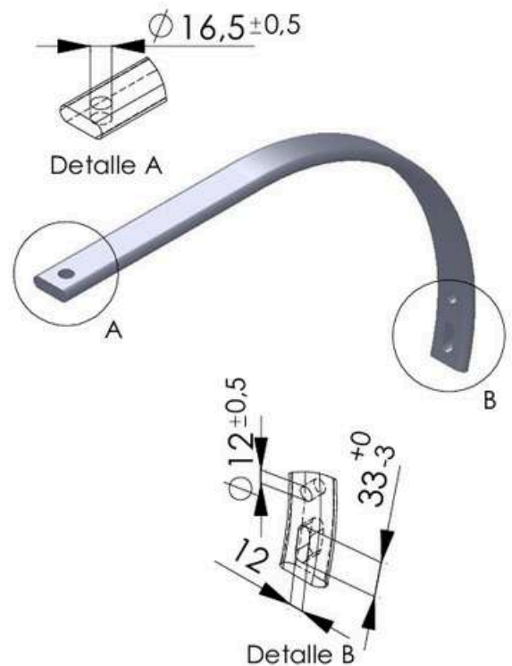
ONAR100 Arcos Tipo "C" Cultivador De Campo
